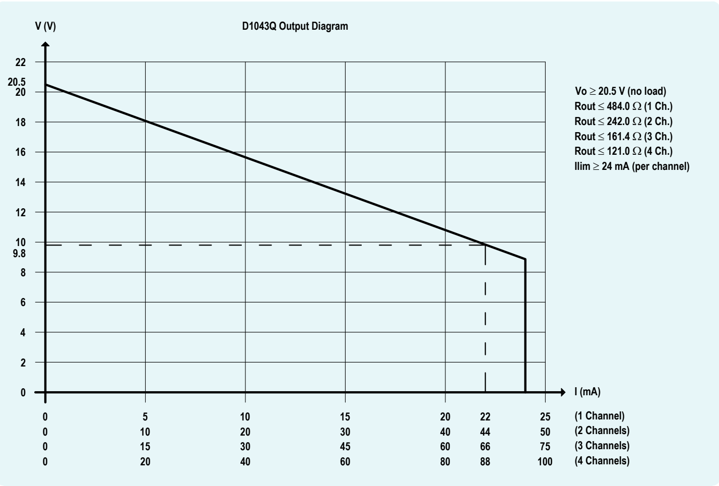
D1043Q OUTPUT DIAGRAM
